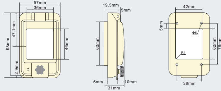
PWW-3 - Dimensions et plan de perçage
