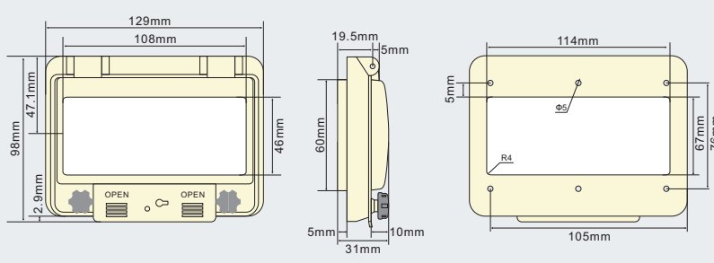
PWW-6 - Dimensions et plan de perçage
