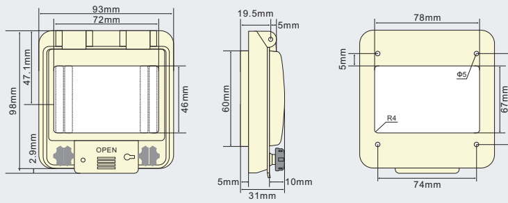
PWW-6 - Dimensions et plan de perçage
