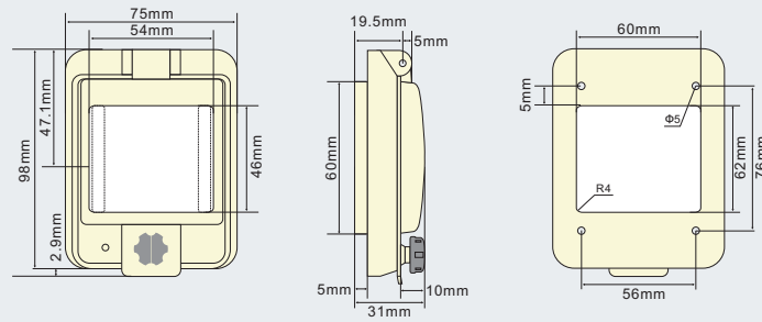
PWW-4 - Dimensions et plan de perçage
