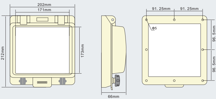
PWW-400K - Dimensiones y orificios de montaje
