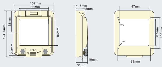
PWW-144K - Dimensiones y orificios de montaje
