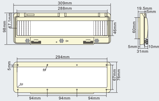
PWW-16 - Dimensiones y orificios de montaje
