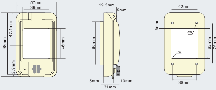
PWW-3 - Dimensiones y orificios de montaje
