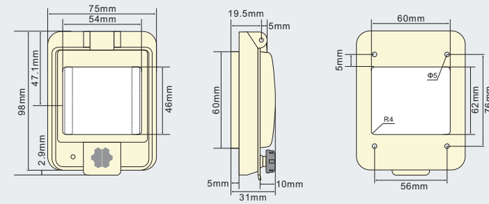
PWW-4 - Dimensiones y orificios de montaje
