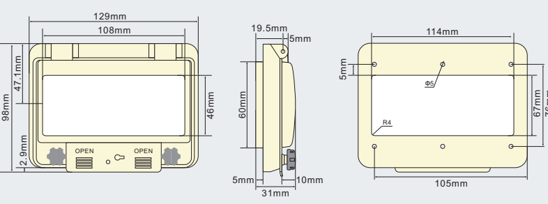
PWW-6 - Dimensiones y orificios de montaje
