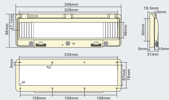
PWW-5 - Dimensiones y orificios de montaje
