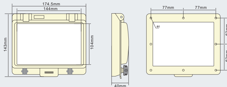
PWW-144K - Dimensiones y orificios de montaje
