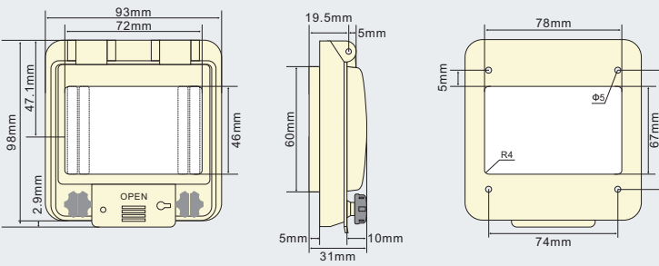
الأبعاد الخارجية وفتحات التثبيت - PWW-6
