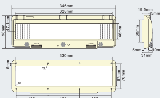
الأبعاد الخارجية وفتحات التثبيت - PWW-5
