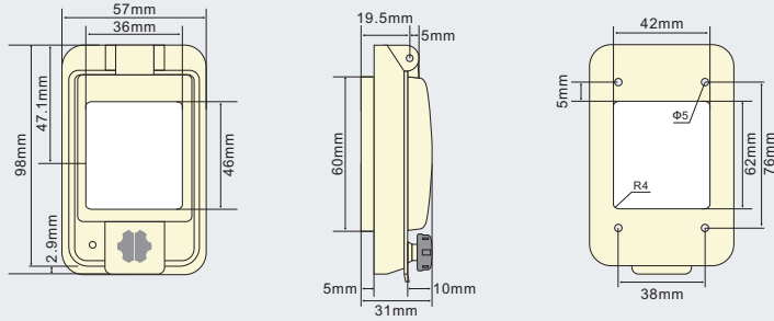
الأبعاد الخارجية وفتحات التثبيت - PWW-3
