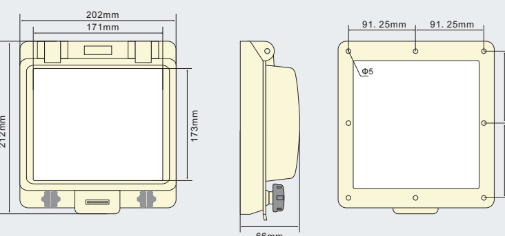
الأبعاد الخارجية وفتحات التثبيت - PWW-400K
