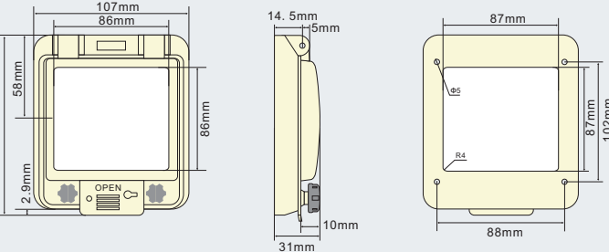
الأبعاد الخارجية وفتحات التثبيت - PWW-144K
