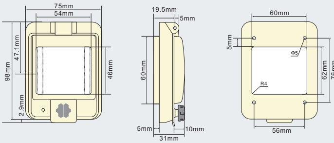
الأبعاد الخارجية وفتحات التثبيت - PWW-4
