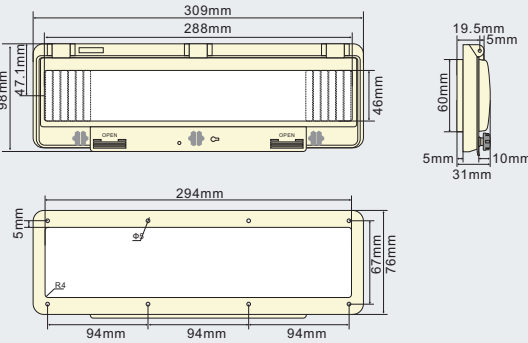
الأبعاد الخارجية وفتحات التثبيت - PWW-18
